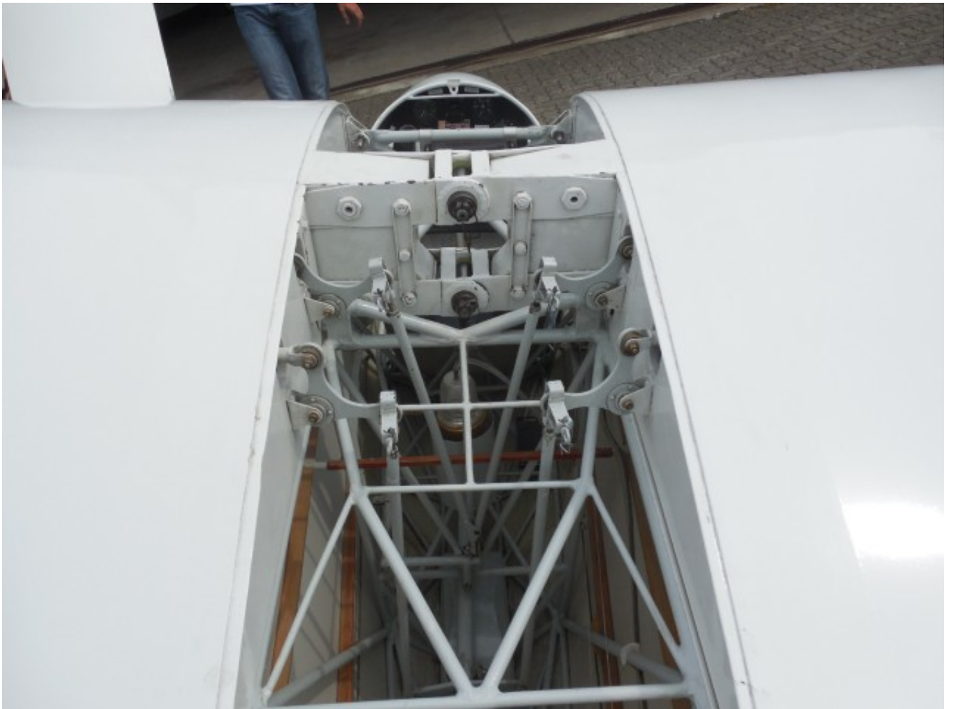
— Blick in den Stahlrohrumpf auf das Rudergestänge.
